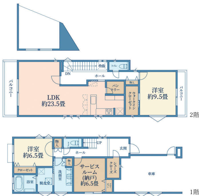
間取図
